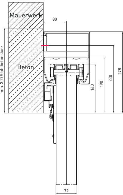
NORMALSTURZ WANDMONTAGE MIT VERDECKTER RAUCHDICHTUNG
