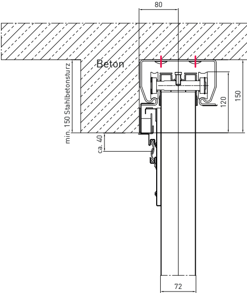
NIEDRIGSTURZ DECKENMONTAGE MIT VORHANDENEM STURZ
