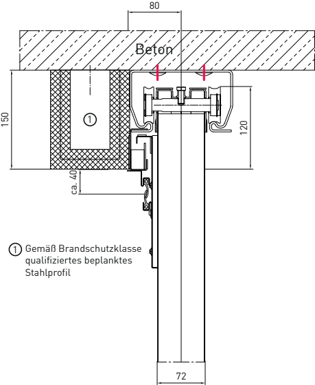
NIEDRIGSTURZ DECKENMONTAGE MIT STURZBLENDE
