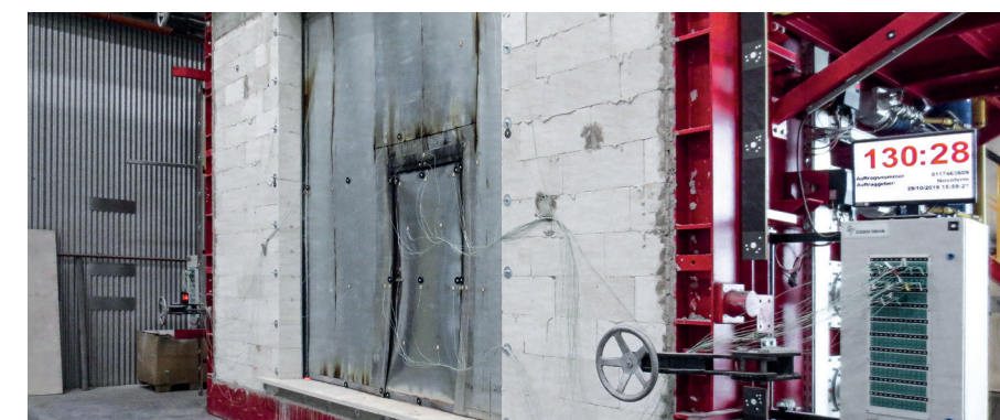
Brandprüfung Toransicht nach 130 Minuten
