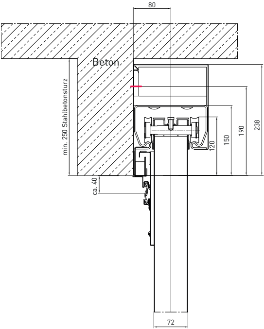
NORMALSTURZ WANDMONTAGE (STANDARD)
