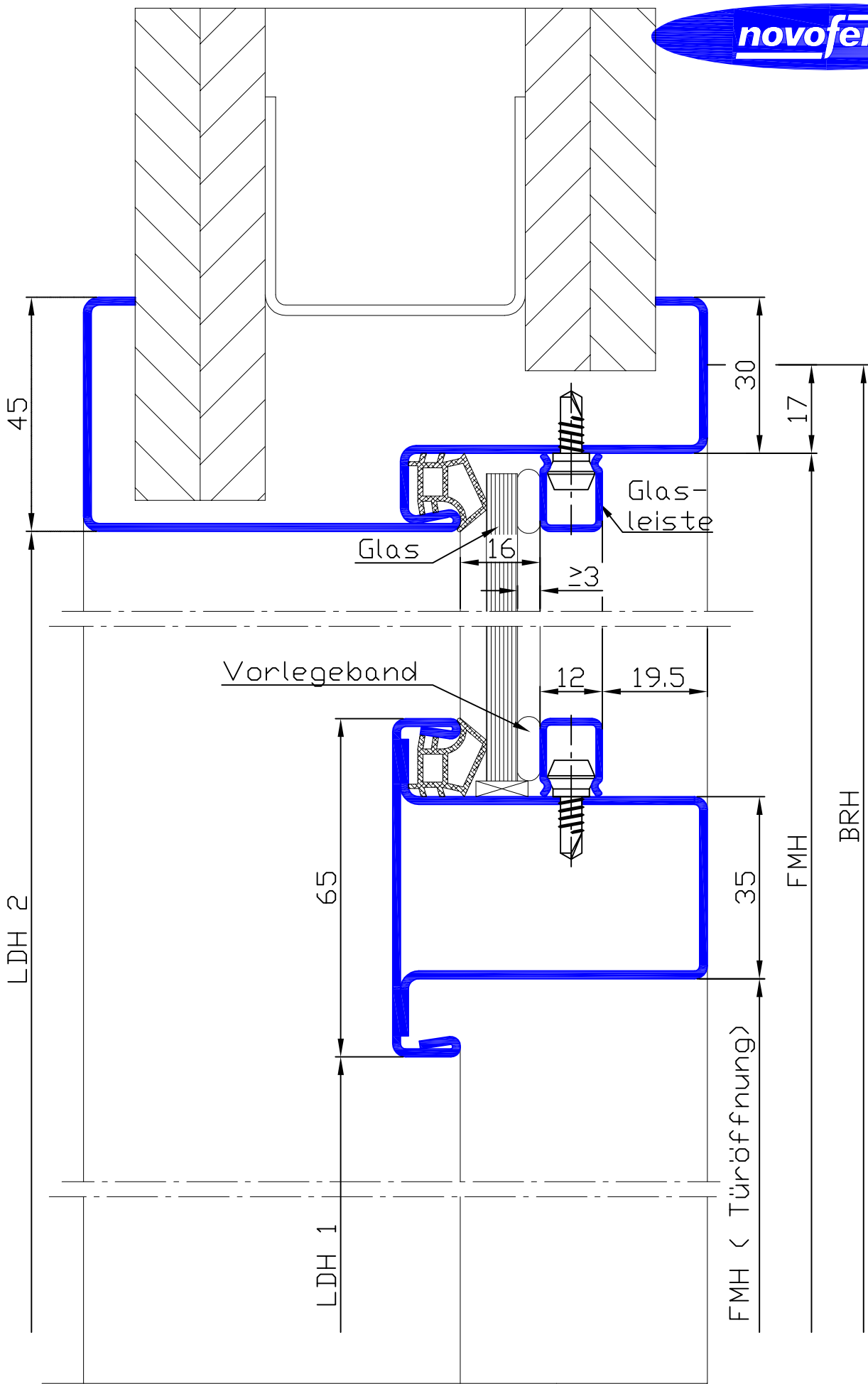
Verglasung und Vorlegeband bauseits
