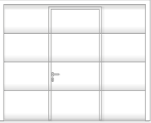
Szimmetrikus elhelyezés középre BRB 2000 - 3500 mm kapuszélességeknél
